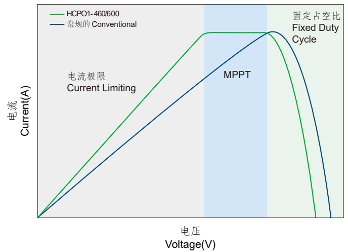
P-V 曲线 P-V Curve
