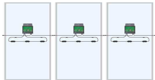
一拖一智能外挂 HCPO1-600 External Optimizer HCPO1-600
