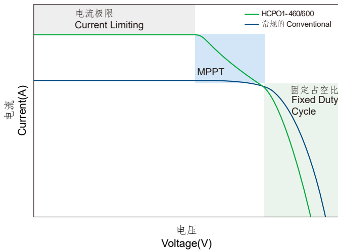
I-V 曲线 I-V Curve
